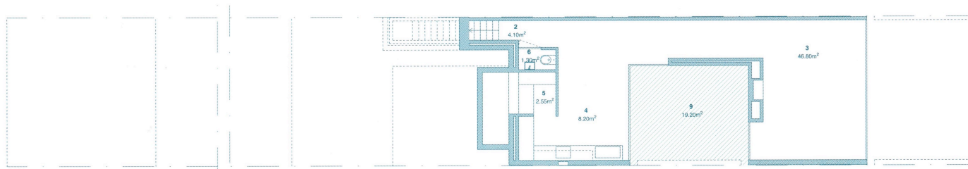
PLANTA DO PISO 0
